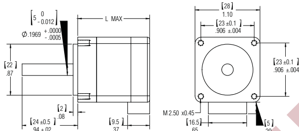
NEMA 11 (28mm)
