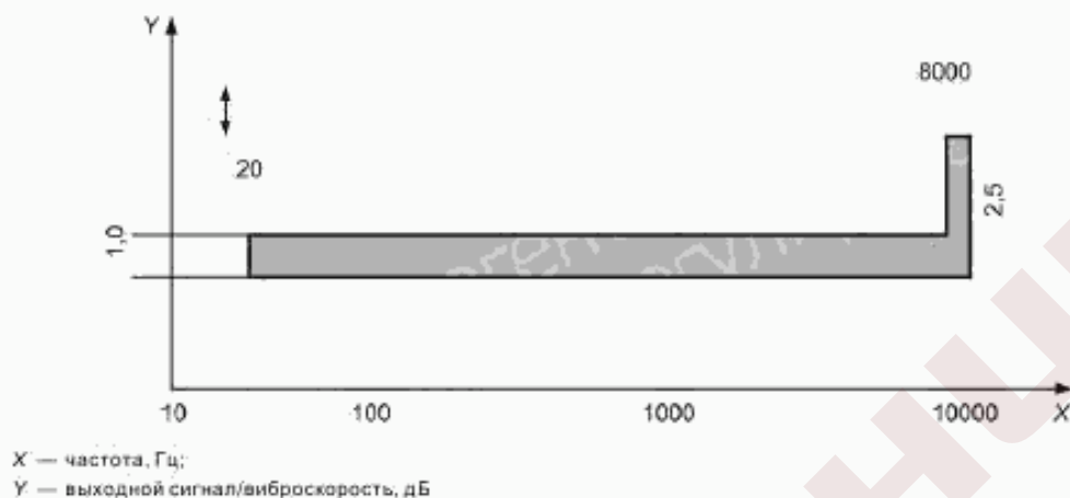
Рисунок 3 — Поле допуска АЧХ вибропреобразователя
